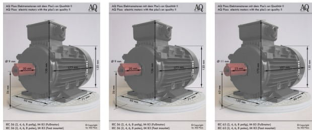
EC Grundformen - Full-Flux-Konstruktion mit ebenfalls möglich EC basic - Assembly - with Full and Flange in possible
