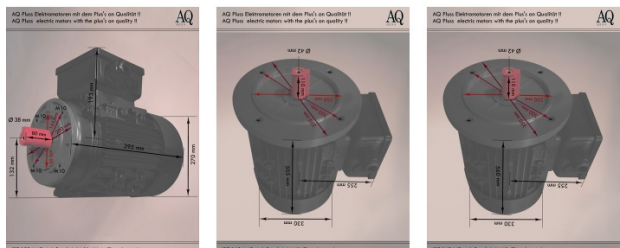
EC 132 M (2, 4, 6, 8 polig), IM B14 (Flange mount) EC 132 M (2, 4, 6, 8 polig), IM B14 (Flange mount) © Copyright by AQ Plus
