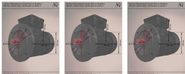
EC 132 M (2, 4, 6, 8 polig), IM B3 (Flange mount) EC 132 M (2, 4, 6, 8 polig), IM B3 (Flange mount) © Copyright by AQ Plus
