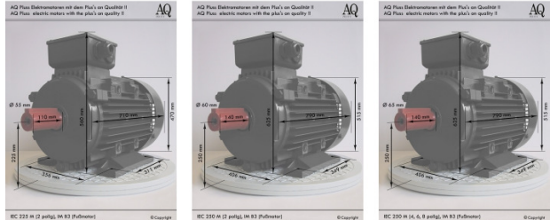
EC 225 M (2 polig), IM B3 (Flanzenmotor) EC 225 M (2 polig), IM B3 (Flanzenmotor) EC 225 M (2 polig), IM B3 (Flanzenmotor)
